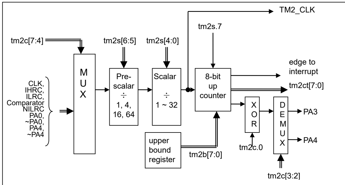
图 13: Timer2 硬件框图
