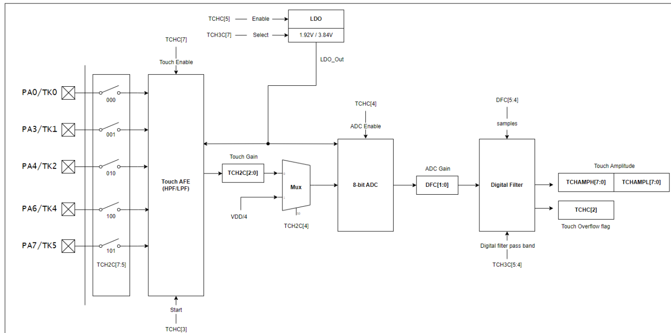
图 23：触摸检测电路的功能方框图
